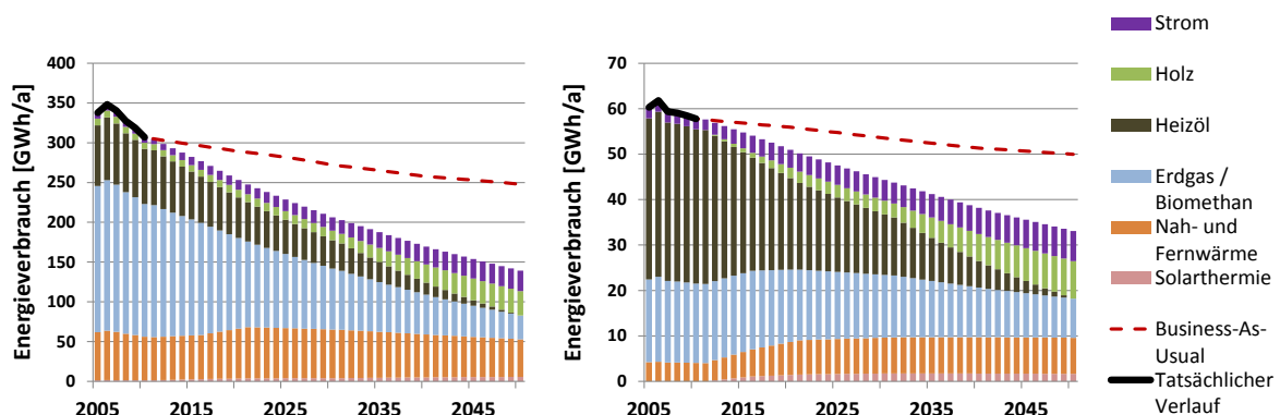
Abbildung 1-4: Entwicklung der Energieversorgungsstruktur im Klimaschutz-Szenario für den Bereich der ehemaligen NEK (links) sowie der ELLM und PEK (rechts)
