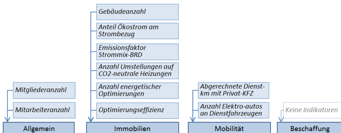
Abbildung 10-3: verwendete Indikatoren
